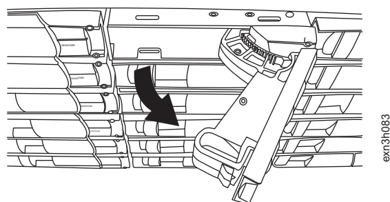
图 9. 卸下磁盘驱动器
