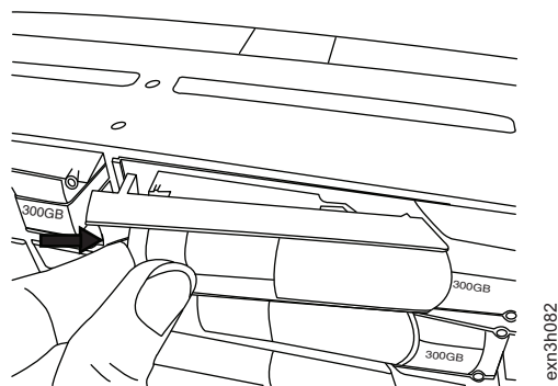
图 8. 松开磁盘驱动器
