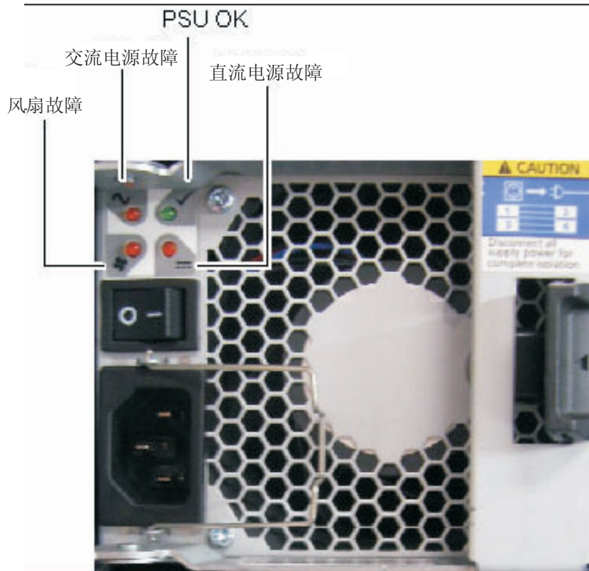
图 7. 电源单元指示灯
