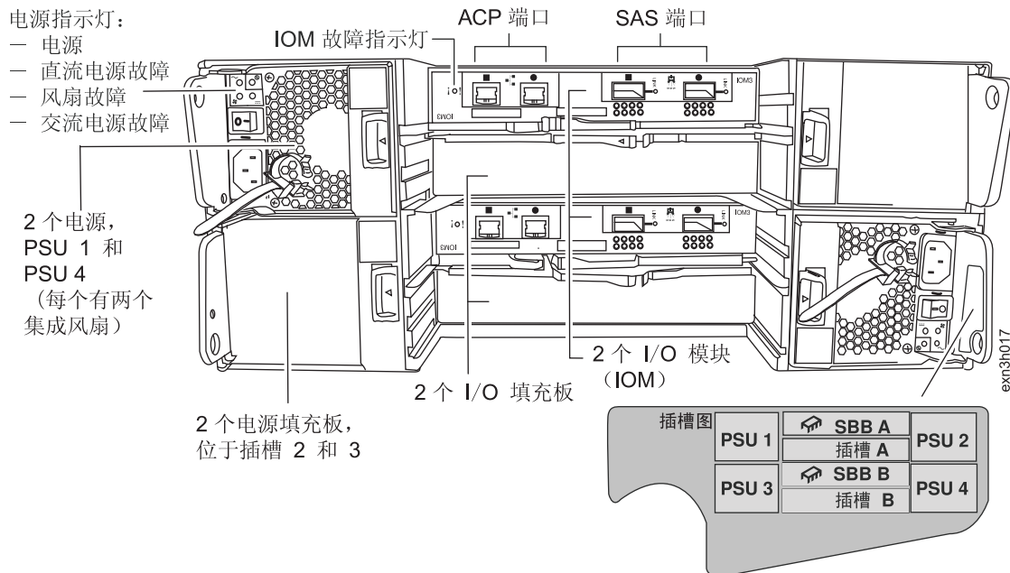
图 2. 具有两个电源的 EXN3000 存储扩展单元的后视图
