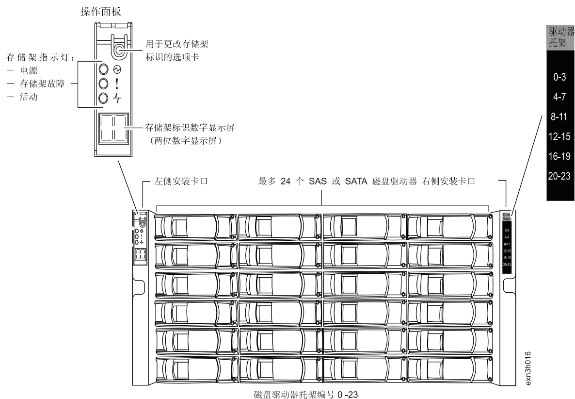
图 1. EXN3000 存储扩展单元的前视图
